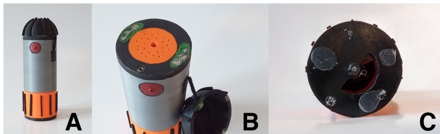
Abbildung 1: (A) Prototyp, (B) Mikrofon, (C) Öffnung an der Unterseite (im drehbaren Aufsatz)
